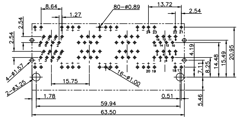
PCB LAYOUT(t=1.60mm)
