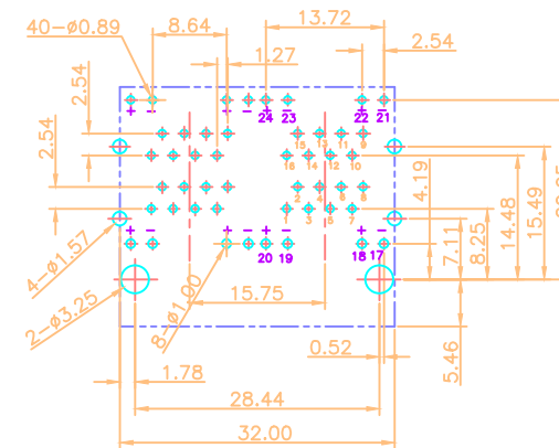
PCB LAYOUT(t=1.60mm)
